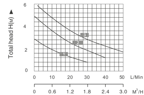
Рабочее поле насосов GRS25/6, GRS32/6, TRS32/6, GRS-SS25/6
