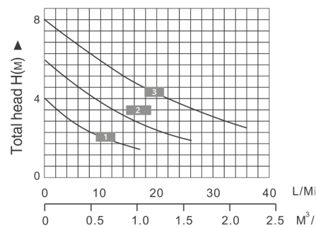
Рабочее поле насосов GRS25/4, GRS32/4, GRS32/4, TRS32/4
