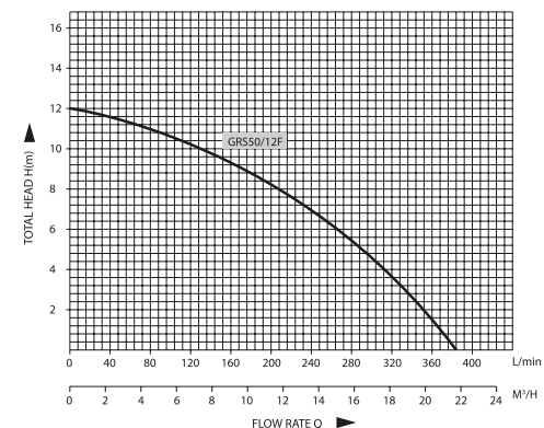
Рабочее поле насоса GRS50/12F
