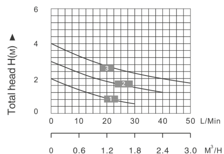
Рабочее поле насосов GRS25/4, GRS32/4, GRS32/4, TRS32/4
