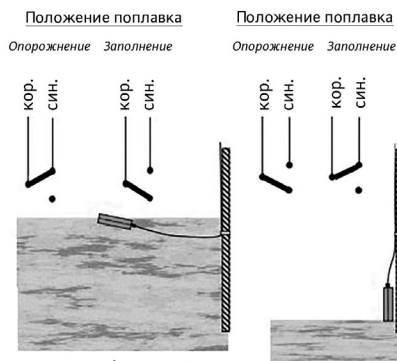
Рис. 4 Электрическое подключение KR 1
