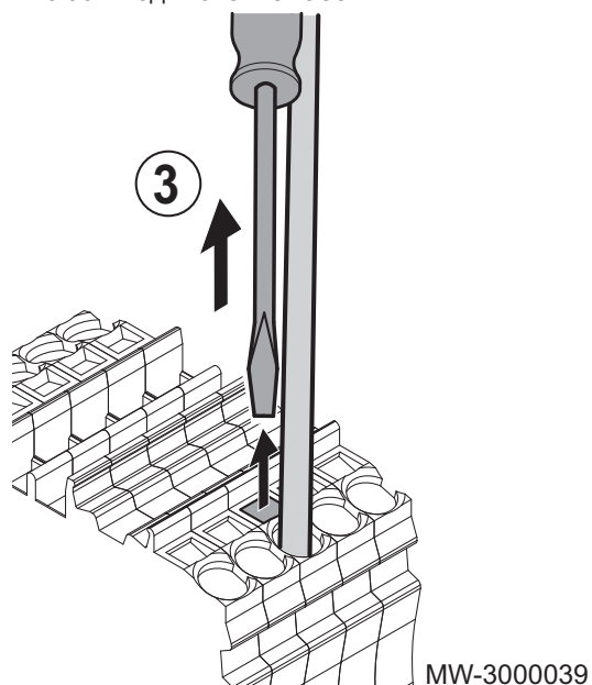
Рис.56 Подключение кабеля
