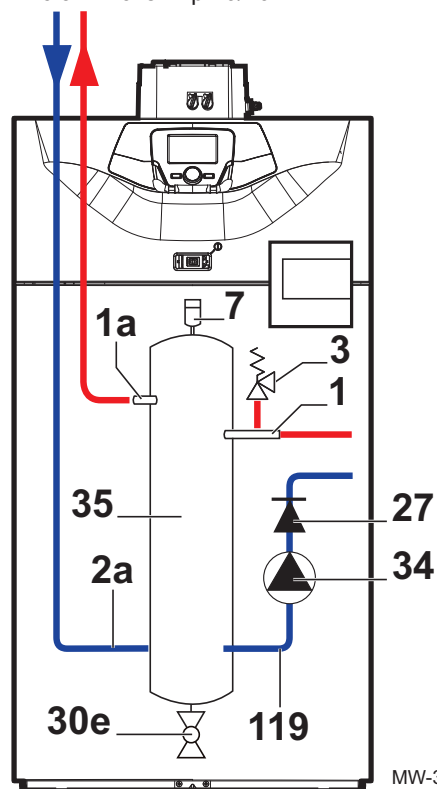
Рис.34 Котел при 0/10 В
