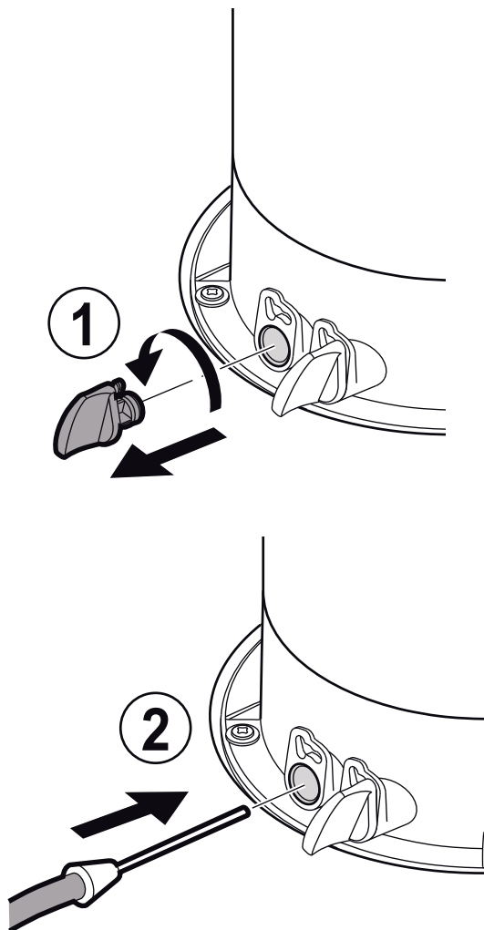
Рис. 146 Подсоединение газоанализатора
