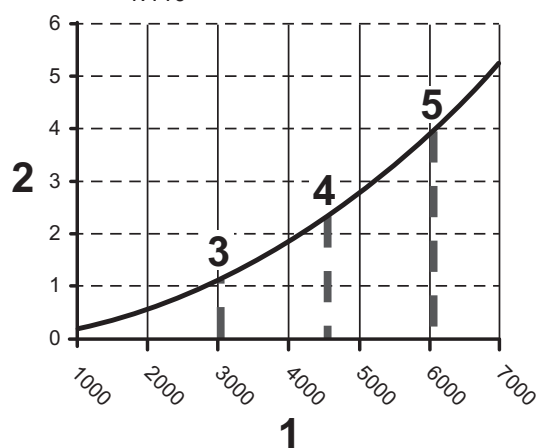
Рис.16 Падения давления для POWER HT + 1.110
