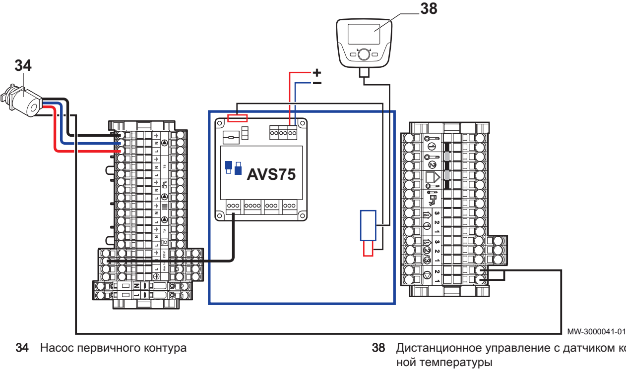
Рис.62 Управление котлом при 0/10 В
