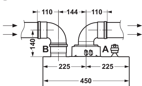
Рис.48 Спецификации раздельных труб для POWER HT+ 1.50 и POWER HT+ 1.70
