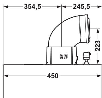
Рис.47 Спецификации коаксиальных труб для POWER HT+ 1.90 и POWER HT+ 1.110
