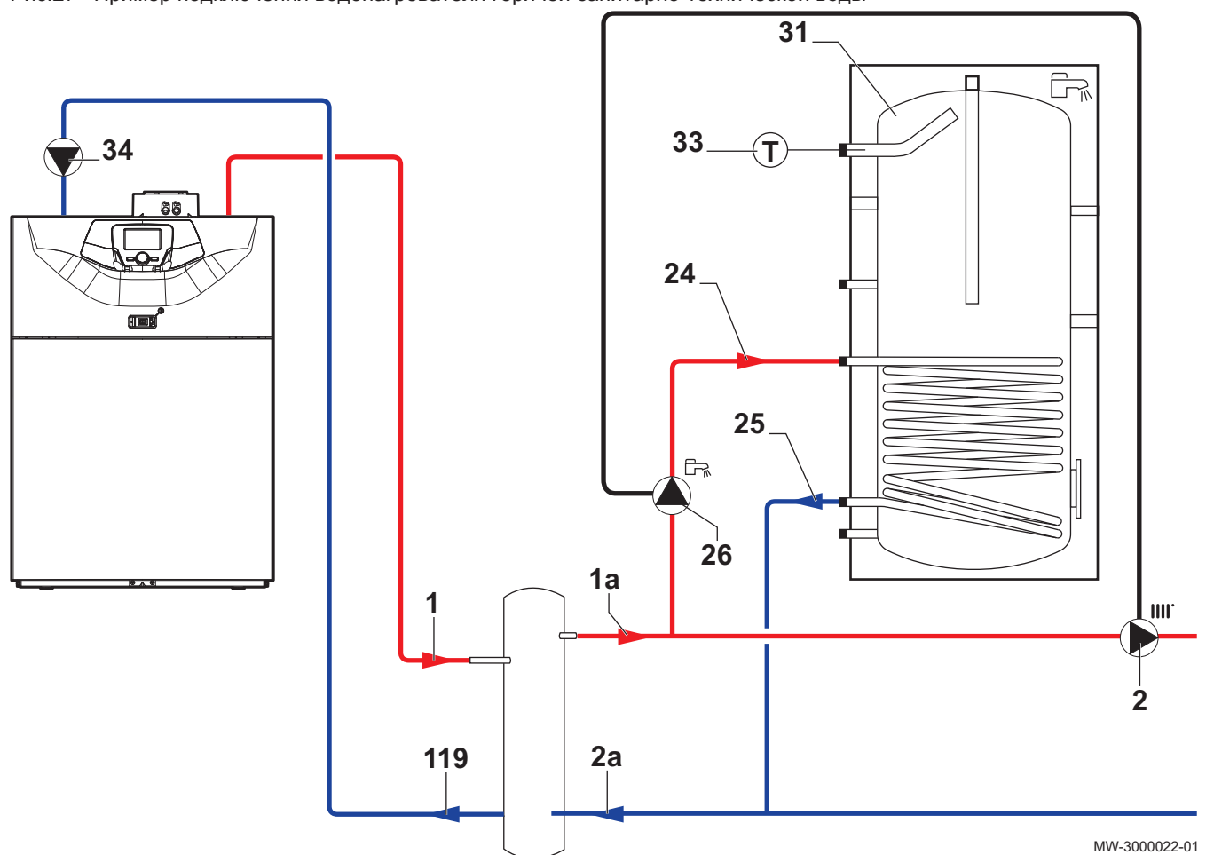
Рис.27 Пример подключения водонагревателя горячей санитарно-технической воды
