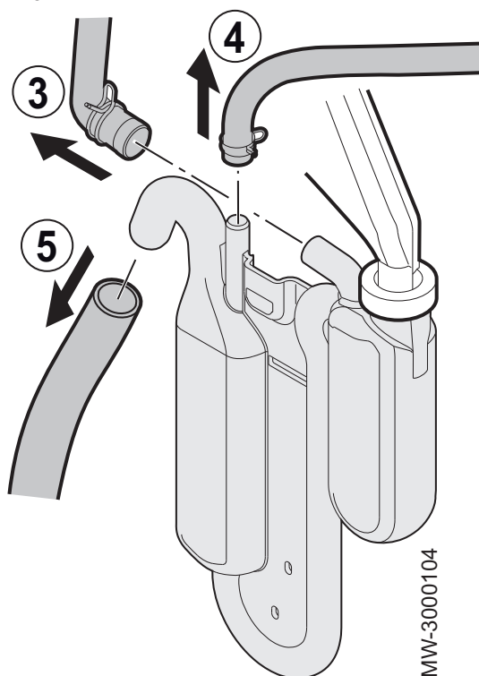
Рис. 145 Снятие сифона
