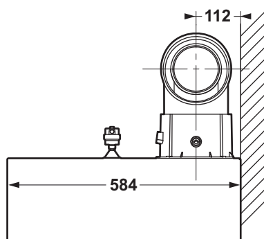
Рис.47 Спецификации коаксиальных труб для POWER HT+ 1.90 и POWER HT+ 1.110
