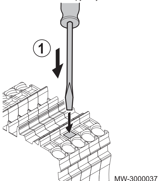
Рис.54 Нажатие на пружину
