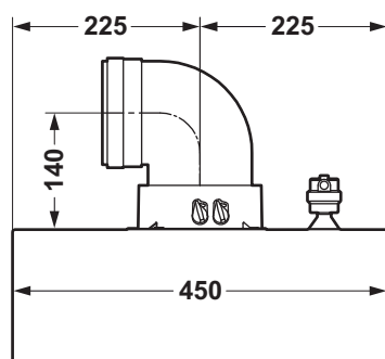
Рис.46 Спецификации коаксиальных труб для POWER HT+ 1.50 и POWER HT+ 1.70
