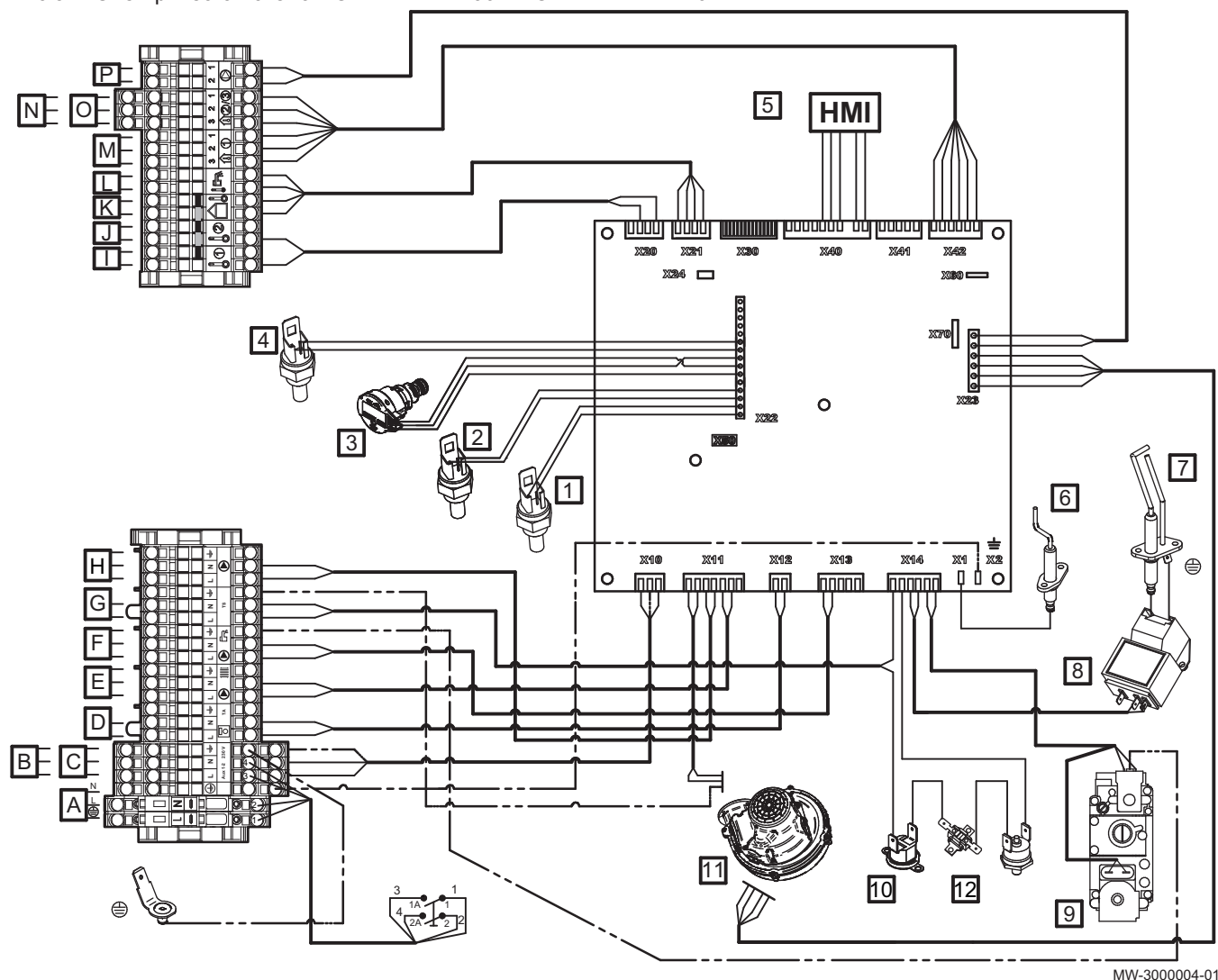
Рис.5 Электрическая схема POWER HT+ 1.90 – POWER HT+ 1.110
