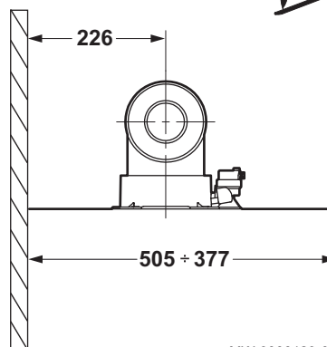
Рис.46 Спецификации коаксиальных труб для POWER HT+ 1.50 и POWER HT+ 1.70
