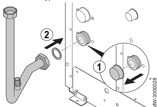
Рис.41 Подключение "подающей трубы контура отопления"
