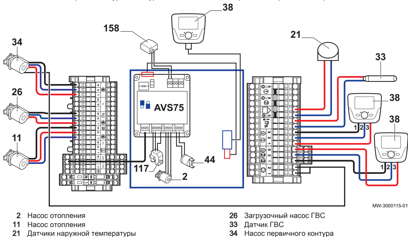
Рис.60 1 котел + 1 прямой контур + 1 контур теплого пола + водонагреватель горячей санитарно-технической воды
