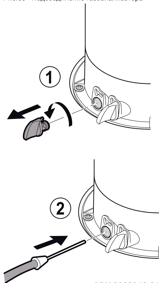
Рис.65 Подсоединение газоанализатора
