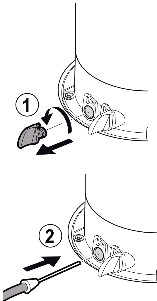
Рис. Подсоединение газоанализатора 148
