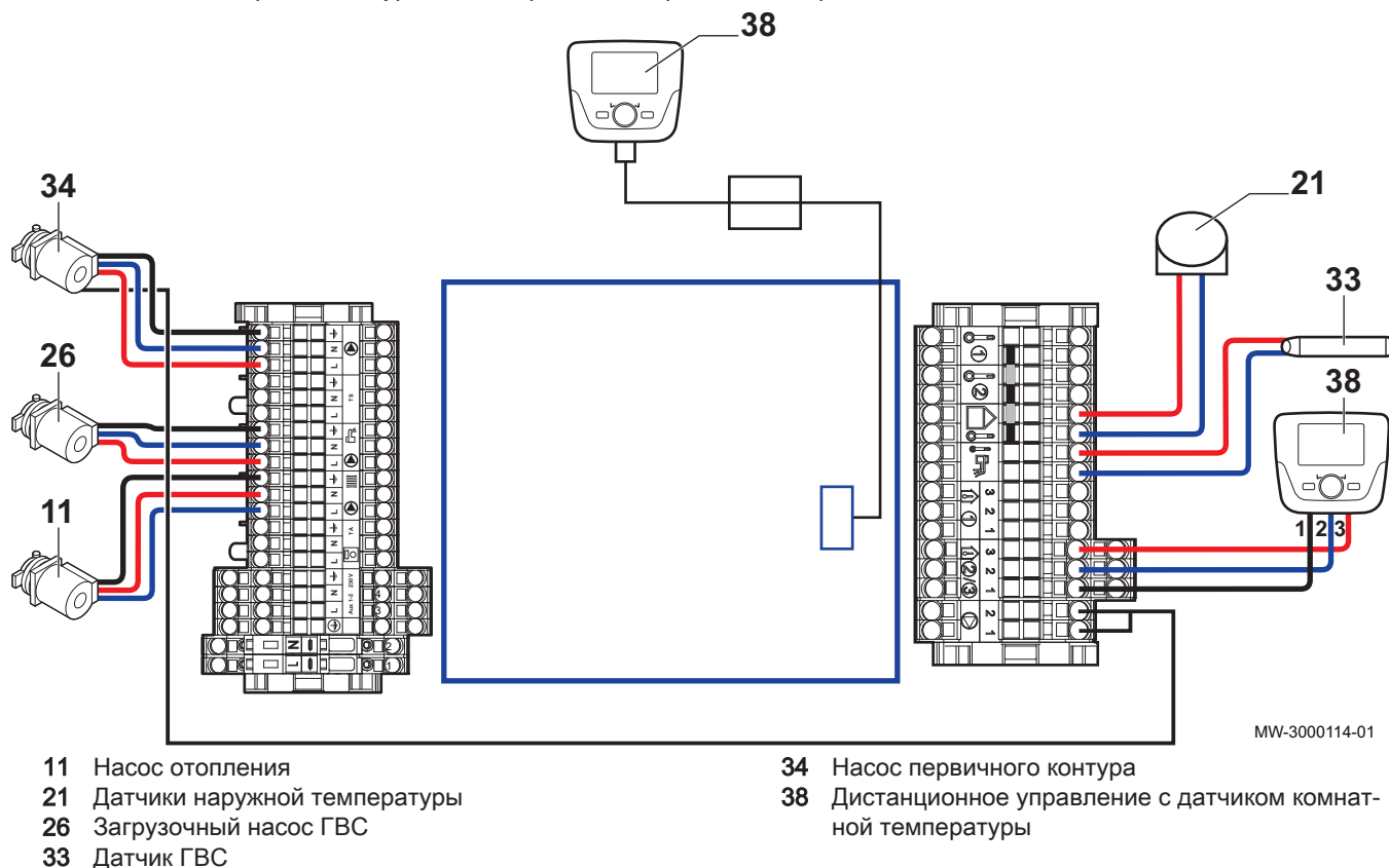
Рис.59 1 котел + 1 прямой контур + водонагреватель горячей санитарно-технической воды
