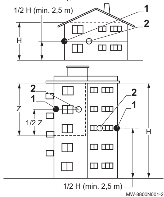
Рис.23 Нерекондуемые места для внешнего датчика
