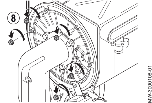
Рис. 138 Снятие удерживающих гаек
