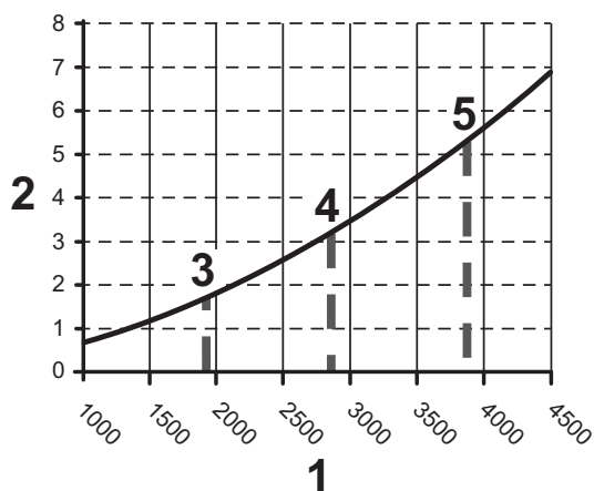
Рис.14 Падения давления для POWER HT + 1.70
