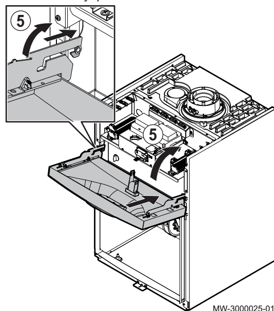
Рис.39 Снятие крышки, закрывающей панель управления
