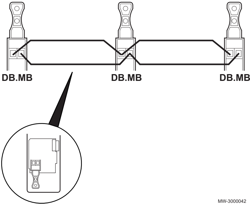
Рис.63 ОЦИ 345 - соединения взаимодействия для каскада
