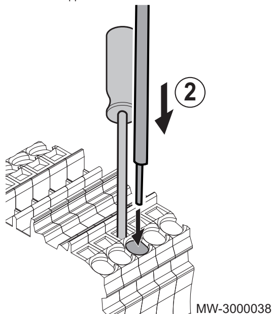
Рис.56 Подключение кабеля
