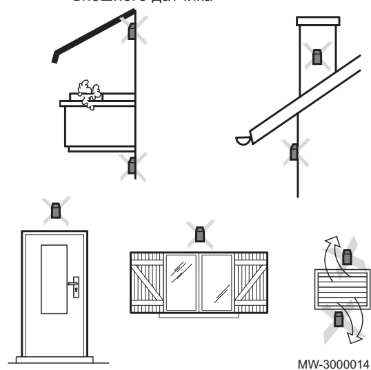
Рис.23 Нерекондуемые места для внешнего датчика
