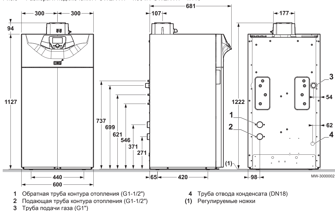
Рис.3 Размеры и подключения POWER HT+ 1.90 и POWER HT+ 1.110
