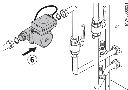
Рис.44 Подключение циркуляционного насоса
