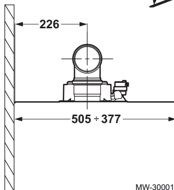
Рис.48 Спецификации раздельных труб для POWER HT+ 1.50 и POWER HT+ 1.70
