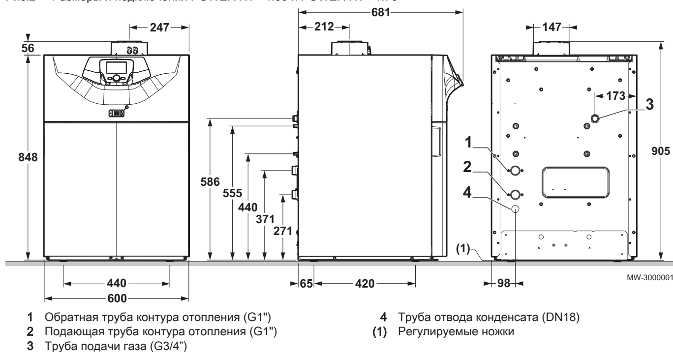
Рис.3 Размеры и подключения POWER HT+ 1.90 и POWER HT+ 1.110
