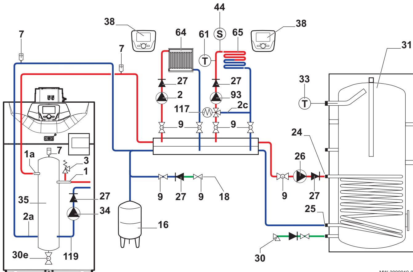
Рис.32 1 котел + 1 прямой контур + 1 контур теплого пола + 1 водонагреватель горячей санитарно-технической воды
