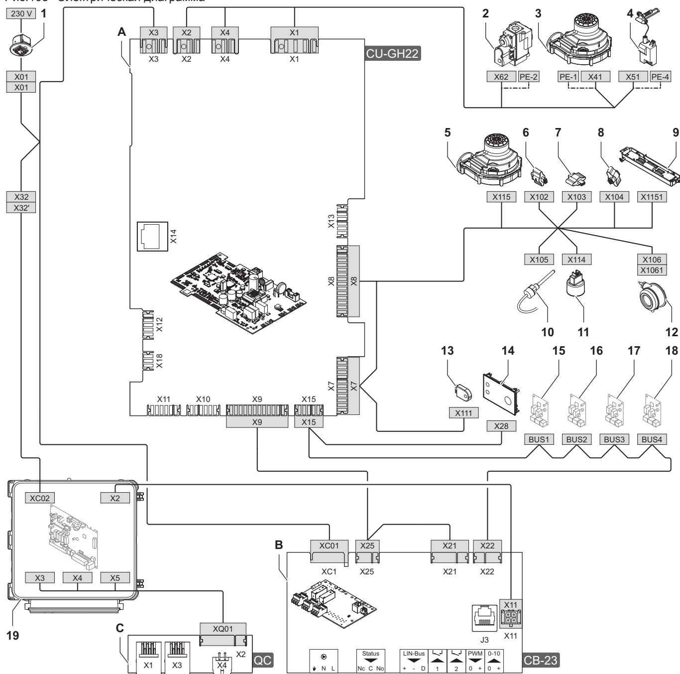
Рис.108 Электрическая диаграмма
