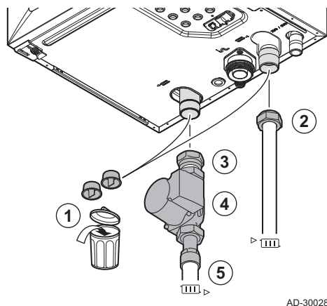
Рис.16 Подсоединение системы отопления
