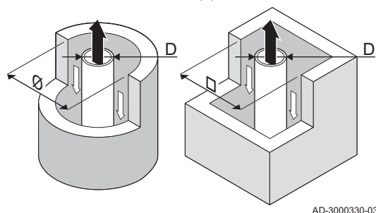
Рис.8 Минимальные размеры шахты или канала C 93(X)
