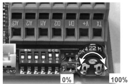
Настройки потенциометра на главной плате
