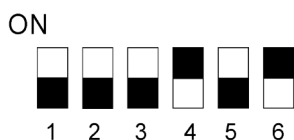
Переключатель DIP, установлен на заводе, Katherm QK/QX, базовая модель C1
