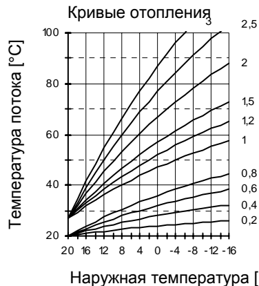
Кривая отопления
