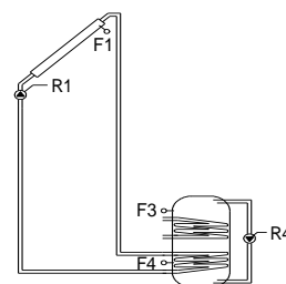
Дополнительная схема с Гидравлической схемой 1
