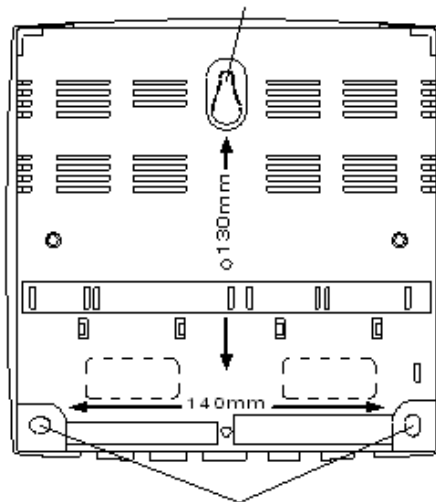
Нижние крепежные отверстия
