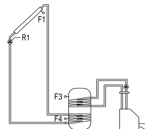
Дополнительная функция показана с Гидравлической схемой 1
