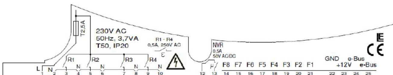
Схема подключений
