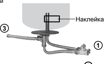
Контрфланец основной ёмкости VG \varnothing 1000 мм и более
