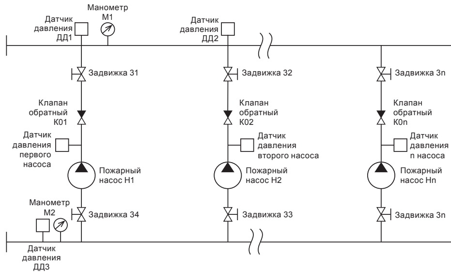
Рис. 9 Общая принципиальная схема установки Hydro-FS-V
