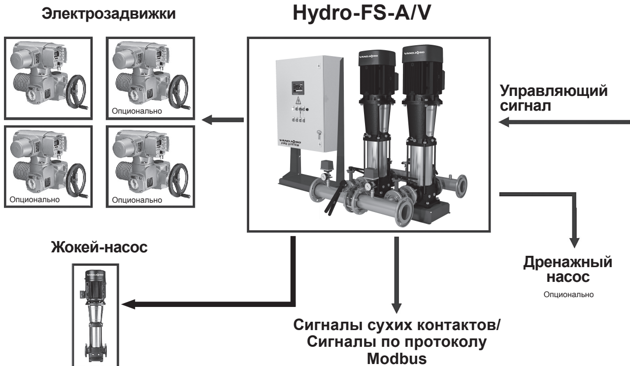
Рис. 11 Общая схема входящих и исходящих подключений
