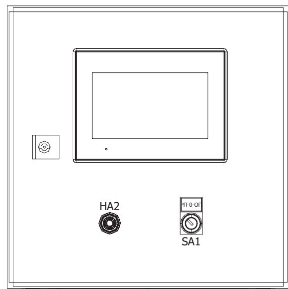
Рис. 12 Удалённая панель диспетчеризации
