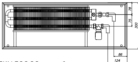
ЕКН.300.90, вид сбоку
