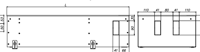
ЕКН.380.200, вид сбоку
