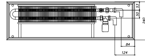
EKN.240.90, вид сбоку
