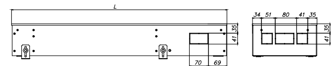
EKN.240.120, вид сбоку
