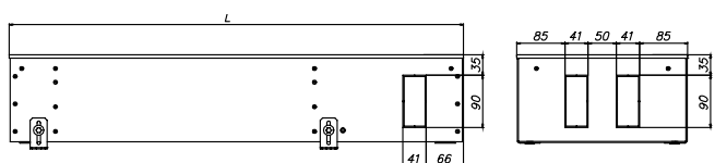
ЕКН.300.200, вид сбоку
