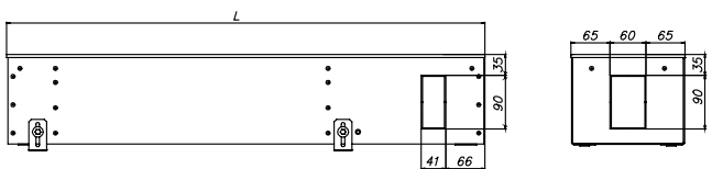
EKN.190.200, вид сбоку
