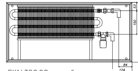
ЕКН.380.90, вид сбоку
