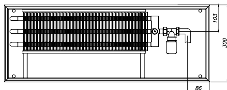
ЕКН.300.150, вид сбоку
