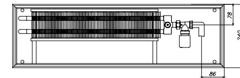
EKN.240.150, вид сбоку
