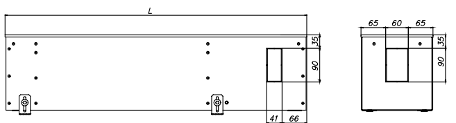
EKN.190.200, вид сбоку
