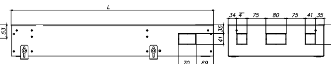
ЕКН.380.150 и ЕКН.380.200, вид сверху
