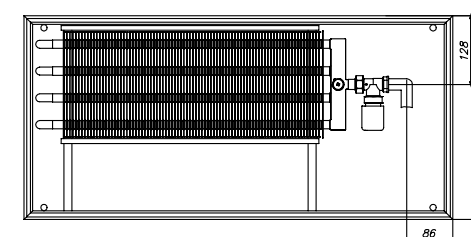
ЕКН.380.150, вид сбоку
