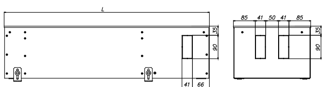
ЕКН.300.200, вид сбоку
