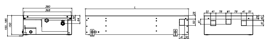
ЕКQ.380.150, вид сбоку
